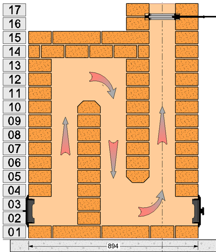
Разрез спереди
