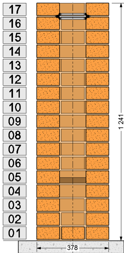
Разрез сбоку
